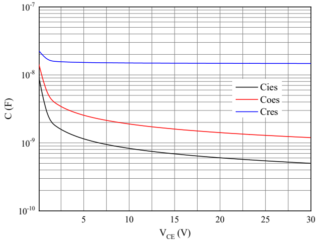
图 9. 电容特性
